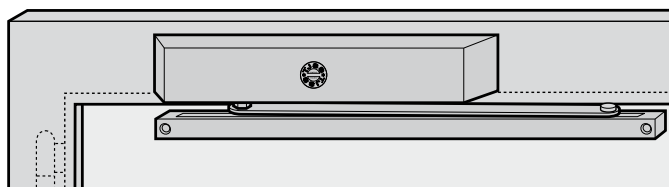
T46: montage inversé côté opposé
