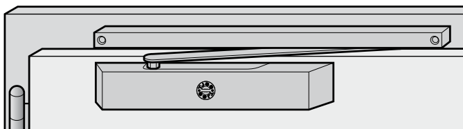
T46: montage normal côté fiché
