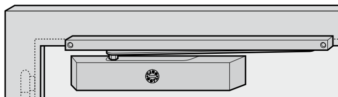
T46G: montage normal côté opposé
